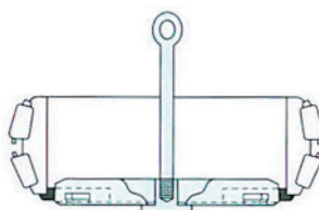
2. Подъемное оборудование для сдвоенного конического сборочного узла подшипника (б)
