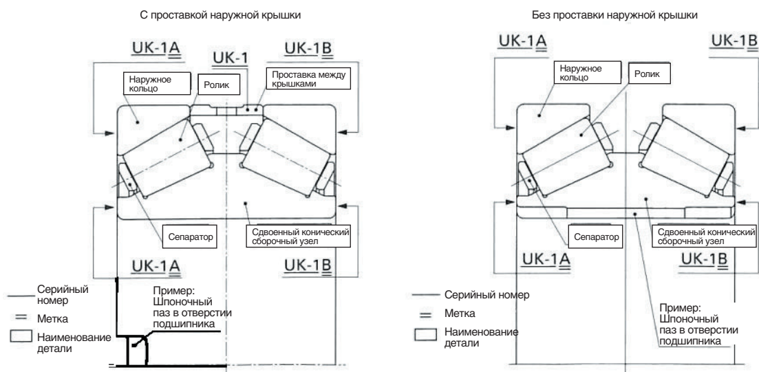
Рис. 1.4 Наименование деталей и примеры маркировки (двухрядный конический роликоподшипник с максимальновозможным углом контакта)
