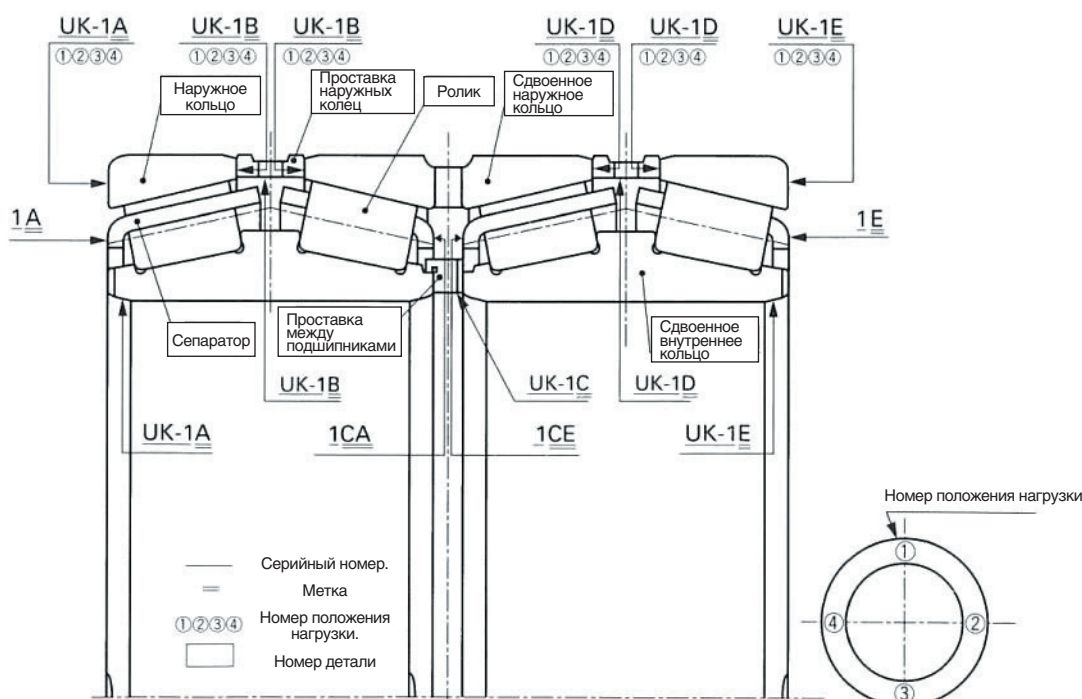
Рис. 1.1 Наименование деталей и примеры маркировки (четырехрядные конические роликоподшипники) Замечание: Некоторые метки могут отсутствовать, если для них недостаточно места.
