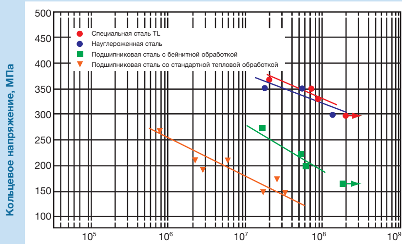
Результаты испытаний на разрушение внутреннего кольца
